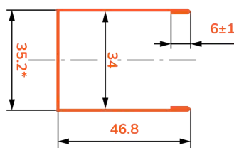
PROFIL "U"
